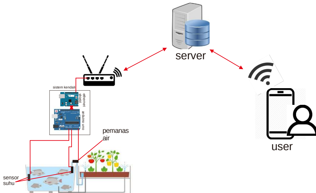
Gambar 1. Arsitektur sensor suhu pada smart aquaponic
